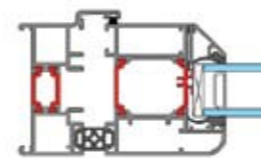
Jamb Detail
